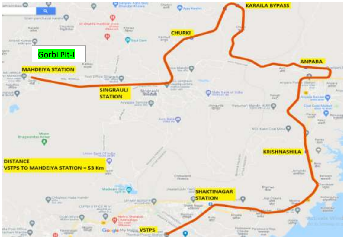
(Gorbi Mine-Void)
